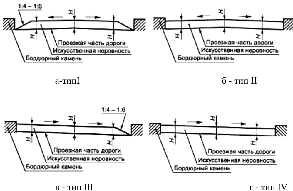
Рисунок 2 - Продольные профили ИН
